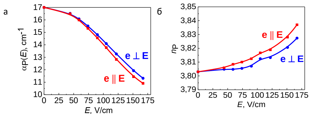
Рисунок 3. Изменения коэффициента поглощения (а) и показателя преломления (б) в InSb n-типа для света с длиной волны 118.8 мкм, поляризованного по полю и против поля.
