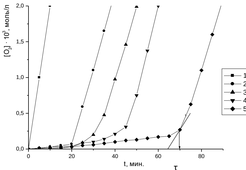
Рисунок 1. Кинетические кривые поглощения кислорода при окислении кумола в отсутствие (1) и в присутствии экстрактов: 0,253 мг СПМ (2), 0,25 мг ВПМ (3), 0,62 мг ВПМ (4) и 0,503 мг СПМ (5). V_i = 1,25 \cdot 10^{-7} моль/л·с, T=348\text{K} .
