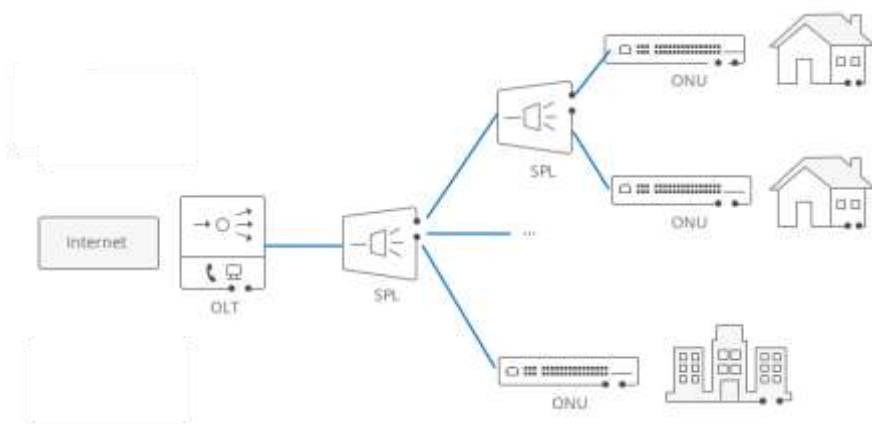
Рисунок 1. Структурная схема проектируемой сети XGS-PON.
