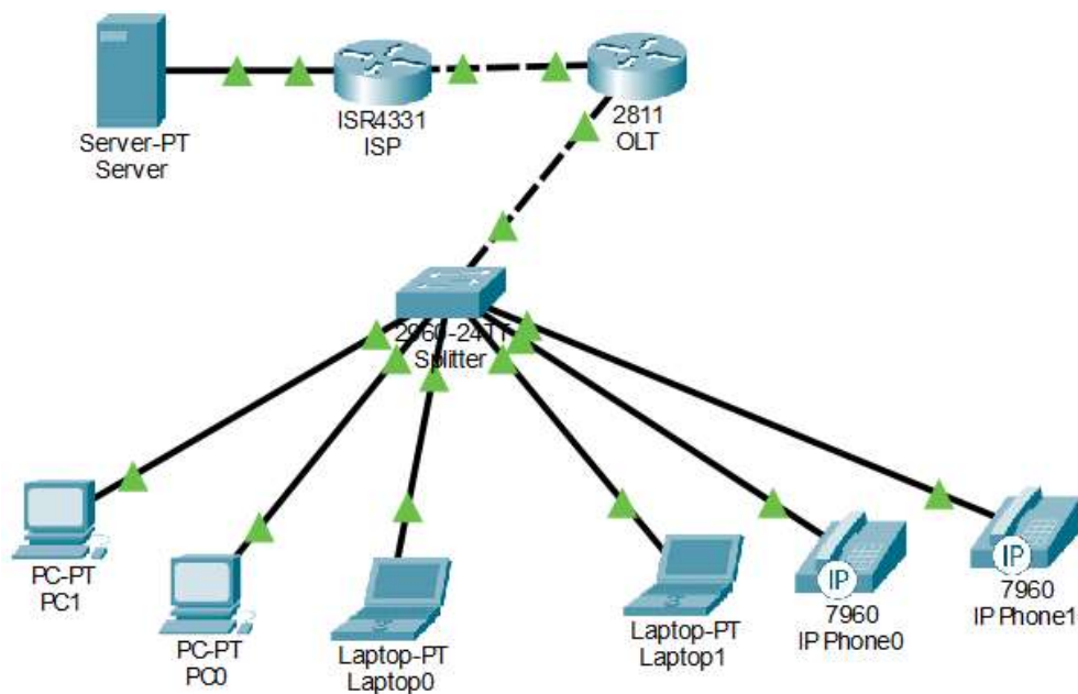
Рисунок 2. Модель проектируемой сети в среде Packet Tracer.
