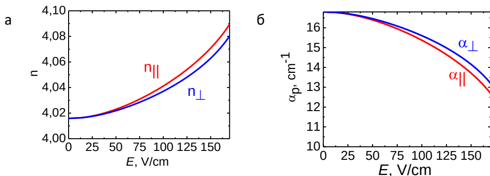
Рисунок 1. (а) Зависимость показателя преломления в InSb от величины приложенного электрического поля для двух поляризации света; (б) Зависимость коэффициента поглощения от величины электрического поля двух поляризаций света.
