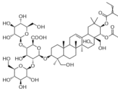
Рисунок 1. Структурная формула эсцина.
