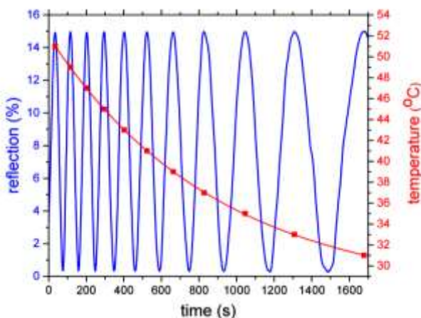
Рис.2. Осциллирующая кривая/левая шкала: временная динамика измеренного отраженного сигнала по мере охлаждения изначально нагретой стеклянной пластины толщиной 15.75мм. Ноль по оси времени соответствует моменту выключения термофена. Экспоненциальная кривая/правая шкала: соответствующее изменение температуры; точки – измеренная температура, сплошная линия – аппроксимация экспоненциальным спадом с постоянной времени \tau = 892.7с .
