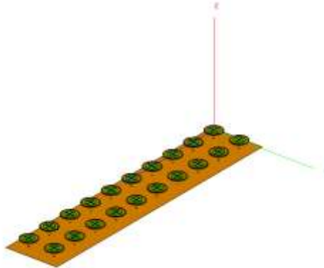
Рис. 4. Модель фазированной антенной решетки.
