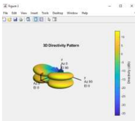
Рис. 3. 3D Диаграмма направленности в MATLAB.
