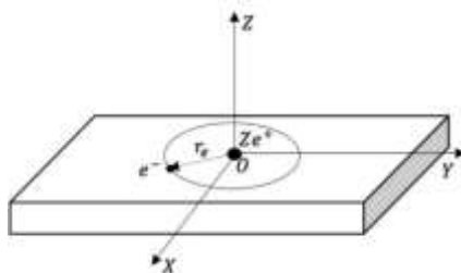
Рис.1. Одновалентная примесь в полупроводниковой нанопластинке.
