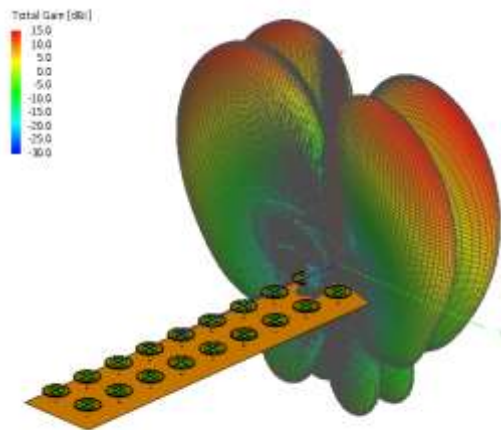
Рис. 5. Результат моделирования.
