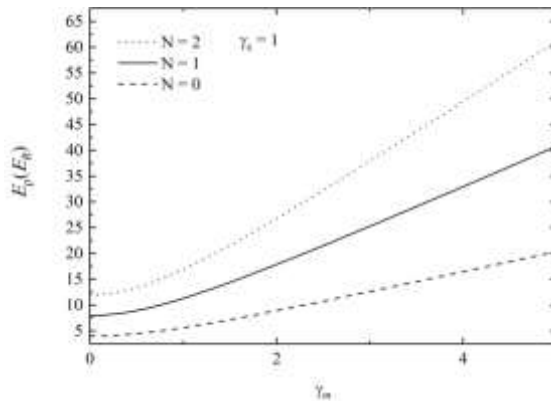
Рис. 1. Зависимость энергии рад.подсистемы от величины магнитного поля для первых трех уровней.
