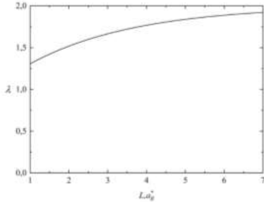
Рис.2. Зависимость вариационного параметра \lambda от L .
