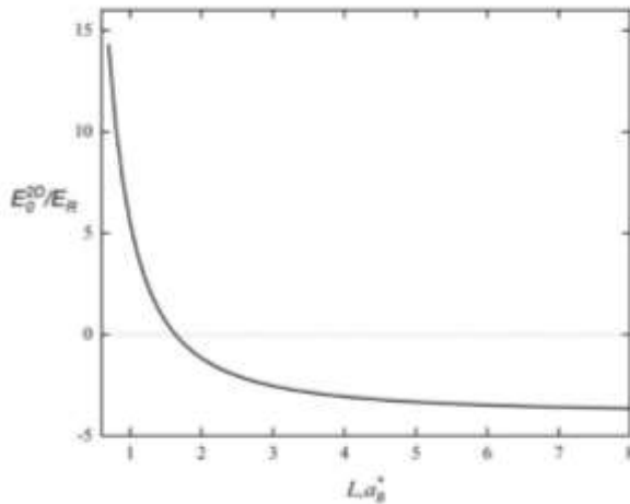
Рис.3. Энергия основного состояния одновалентной примеси в зависимости от L .
