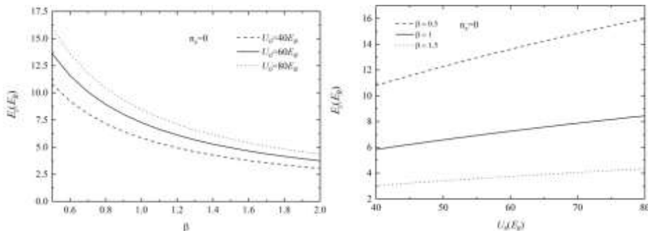
Рис. 2. Зависимость аксиальной энергии от полуширины (а) и глубины (б) МППТ.
