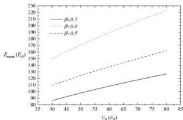
Рис. 4. Зависимость минимальной аксиальной энергии системы от глубины потенциальной ямы при фиксированных значениях ширины потенциальной ямы.
