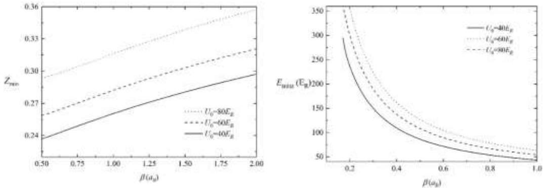
Рис. 3. Зависимость минимального значения z_{\min} (а), а также аксиальной энергии основного состояния биекситона (б) от ширины потенциальной ямы при фиксированных значениях глубины потенциальной ямы.
